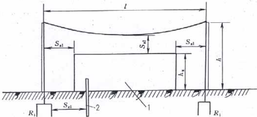
图 4.2.1 防雷装置至被保护物的间隔距离
