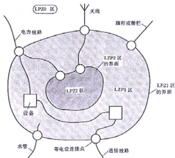
图 15 将一个需要保护的空间划分为不同防雷区的一般原则
