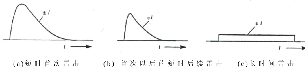
图 F.0.1-1 闪电中可能出现的三种雷击
