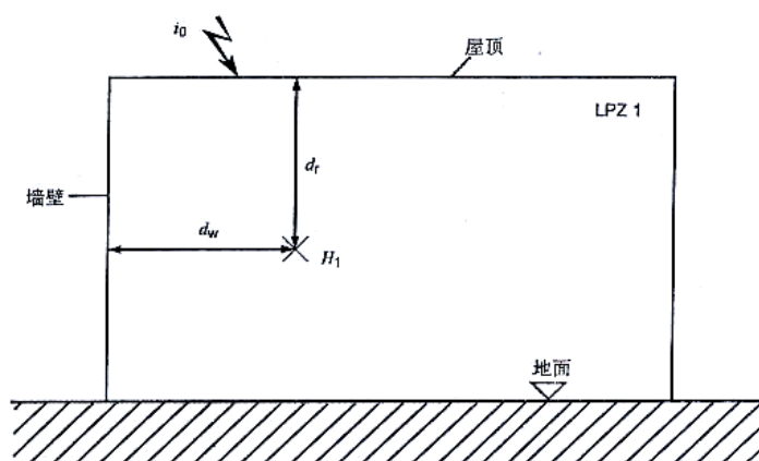
图 6.3.2-4 闪电直接击于屋顶接闪器时 LPZ 1 区内的磁场强度 (6.3.2-8) 式的计算值仅对距屏蔽格栅有一安全距离的安全空间内有效，安全距离应按下列公式计算。
