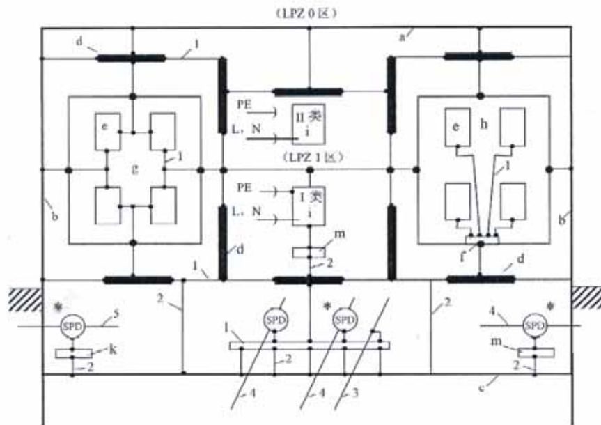
图 6.3.3 接地、等电位连接和接地系统的构成
