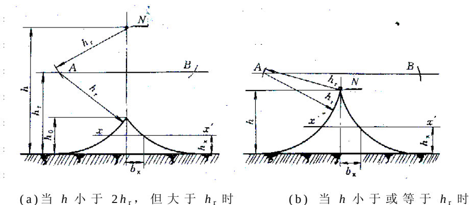
图 D.0.5 单根架空接闪线的保护范围
