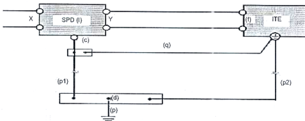
图 J.2.4-2 将多接线端子电涌保护器的有效电压保护水平减至最小所必需的安裝条件的例子
