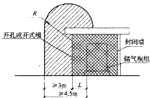
图 C.0.14 存放 CNG 储气瓶(组)的房间爆炸危险区域划分
