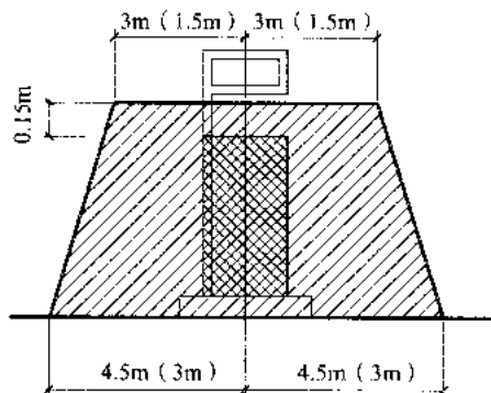
图 C.0.5 汽油加油机爆炸危险区域划分
