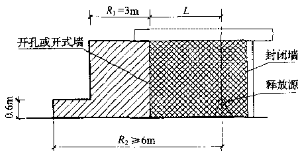
图 C.0.10 LPG 压缩机、泵、法兰、阀门或类似附件的 房间爆炸危险区域划分
