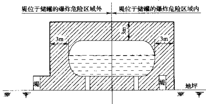
图 C.0.16-1 地上 LNG 储罐的爆炸危险区域划分
