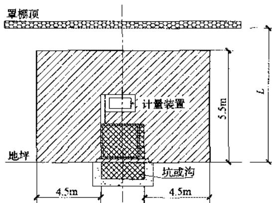
图 C.0.15-1 CNG 和 LNG 加气机的爆炸危险区域划分(一)
