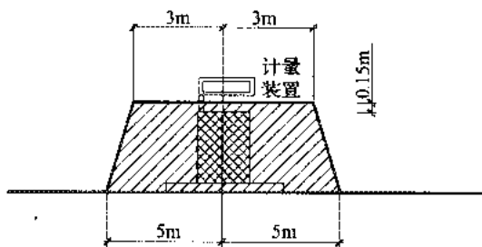
图 C.0.6 LPG 加气机的爆炸危险区域划分
