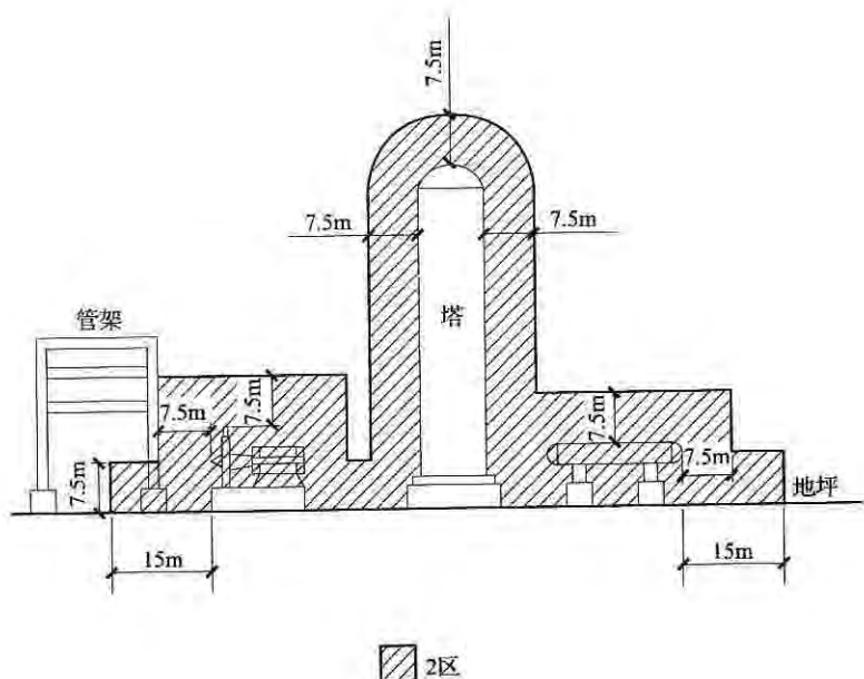
(b) 立面图
